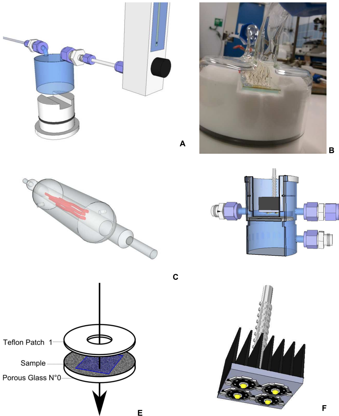
Figure 14 : Schéma des différents réacteurs conçus en fonction de la morphologie des matériaux de fibres de \text{TiO}_2 . A : schéma du réacteur à flux léchant pour les matériaux déposés sur lame de verre ou pour les fibres agencées en « tapis de fakir ». B : photographie des fibres agencées en « tapis de fakir » en place dans le réacteur à flux léchant. C : réacteur à flux léchant pour les fibres (en rouge) agencées dans un capillaire. D : réacteur à flux traversant utilisé pour les fibres de 3 o génération, tissées ou agencées en pelote. E : support pour les fibres de 3 o génération tissées. F : source lumineuse UVA haute puissance développée pour le réacteur à flux traversant.
