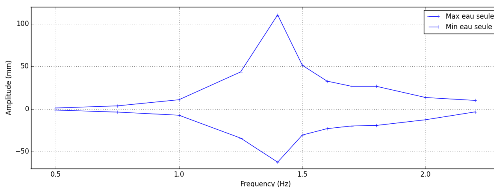
FIGURE 4.23 – Cas du réservoir contenant uniquement 40cm d'eau : amplitude du mouvement de la surface libre en fonction de la fréquence d'excitation.
