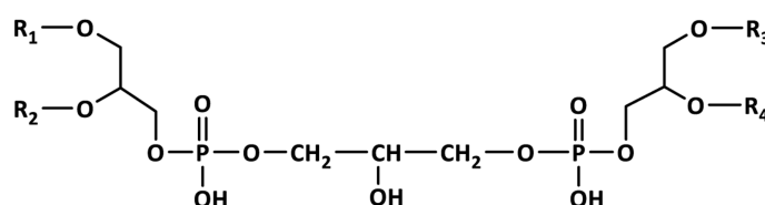
Cardiolipin (CDL)
