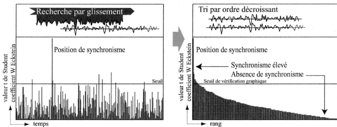
Fig. 62 - Recherche de synchronisme par glissement (graphique O. Girardclos et C. Perrault – Cedre)
