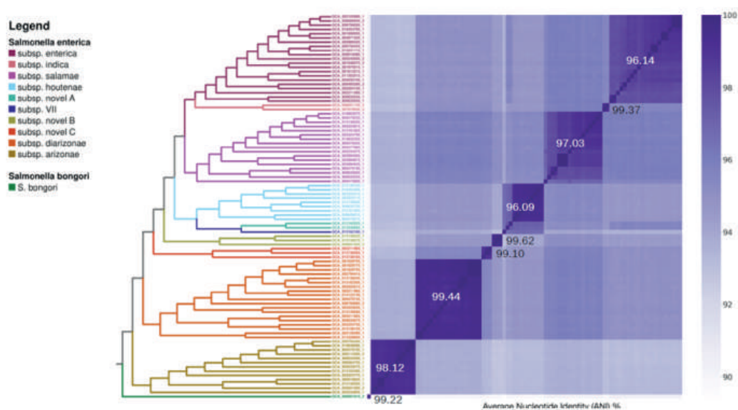
Figure 6. Phylogénie de vraisemblance maximum et carte de chaleur des valeurs d'identité nucléotidique moyenne (ANI) des génomes de Salmonella .
