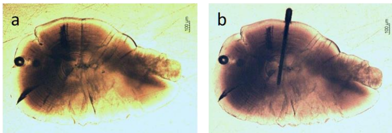
Figure 5 : Photographie d'un otolithe (a) avant et (b) après ablation laser.
