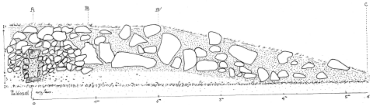
Fig7. Vue en coupe
