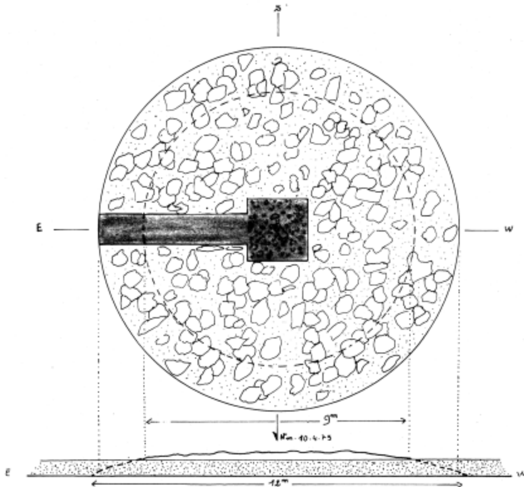
Fig.6. Vue en plan du monument. En grisé, zone exploré.
