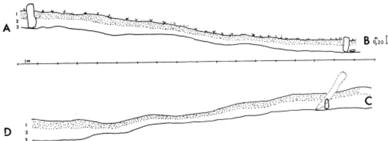
Fig. 3. Les coupes AB et CD mettent en évidence l'inclinaison des sols du terrain vers le nord. Noter que pour plus de clarté l'échelle des abscisses est différente de celle des ordonnées.
