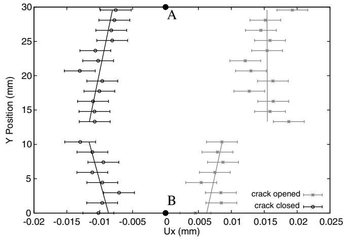
Fig. 19. Horizontal displacements
