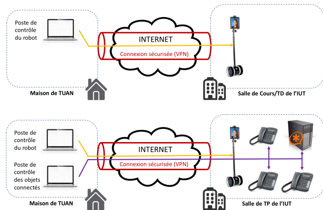
Figure 2 : Architecture de l'environnement pédagogique connecté (en haut, salle de cours / TD ; en bas, salle de TP)
